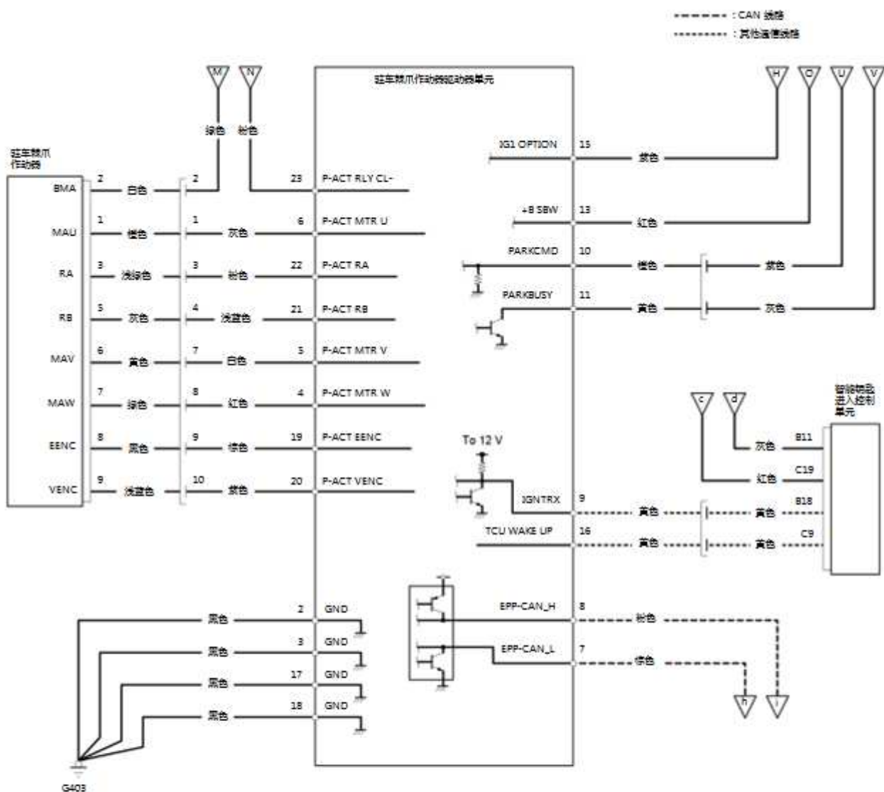
驻车制动执行器控制单元 26 针插接端子位置
